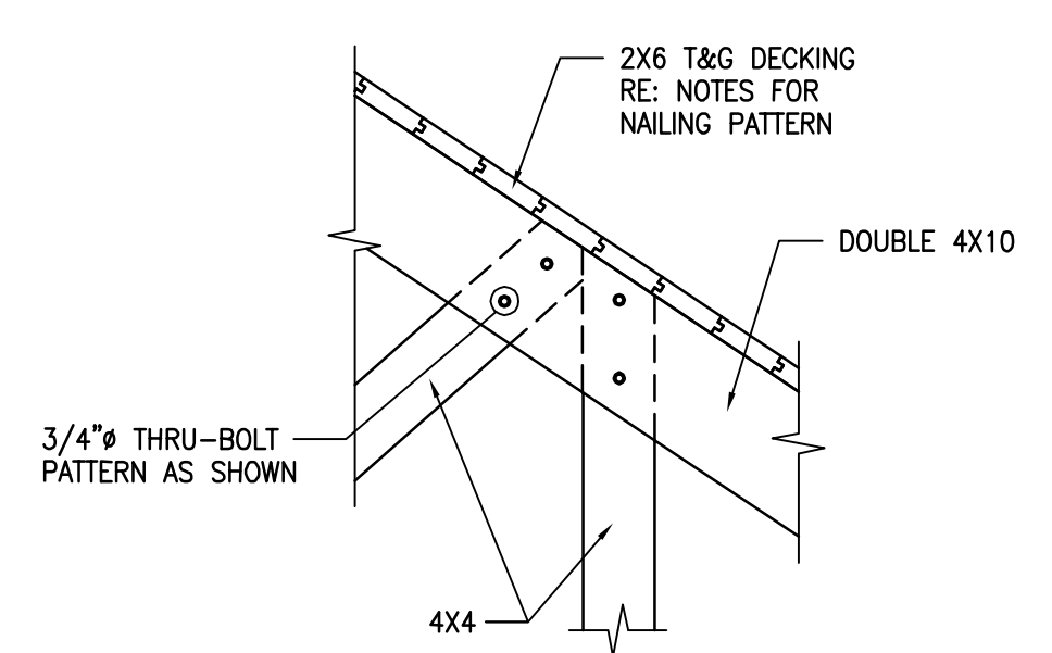
03 SECTION SCALE: 3/4" = 1'-0"
