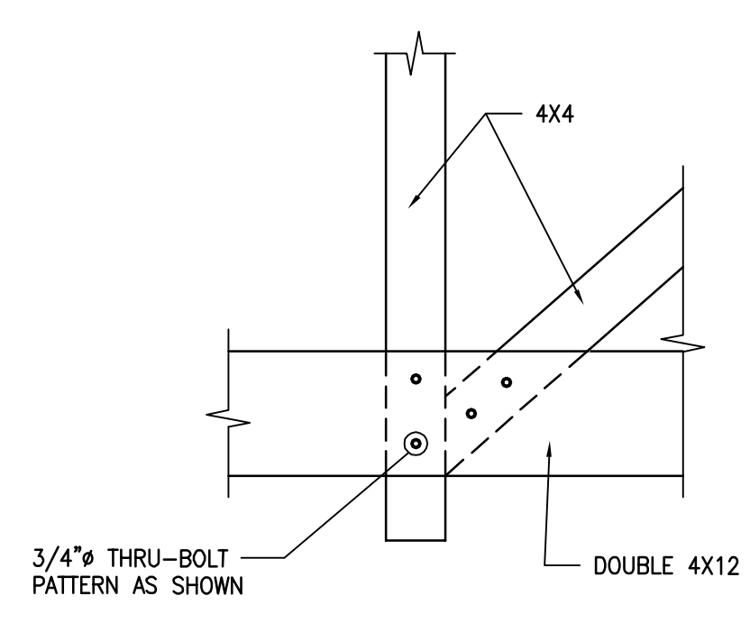
02 SECTION SCALE: 3/4" = 1'-0"
