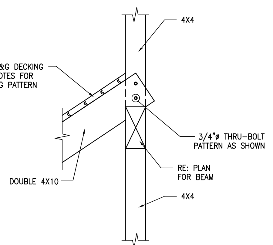
05 SECTION SCALE: 3/4" = 1'-0"
