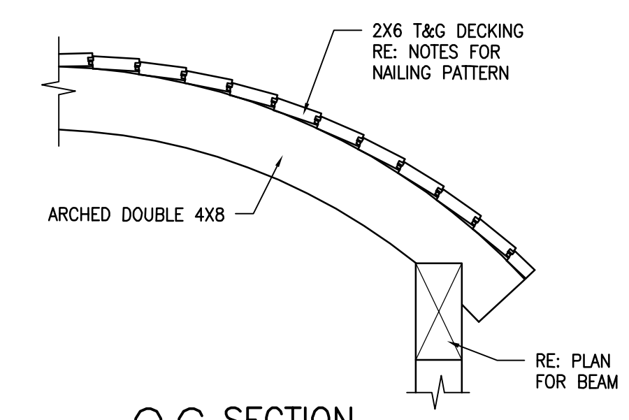
06 SECTION SCALE: 3/4" = 1'-0"
